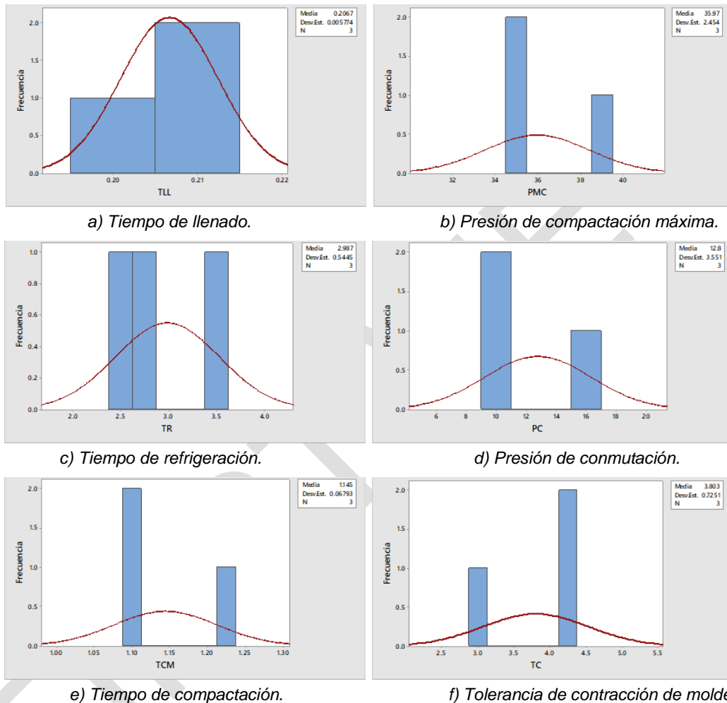
Figura 4 Histogramas para la simulación del buje. Fuente: elaboración propia
