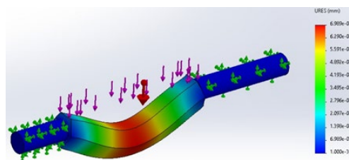
Figura 14 Deformación del eje.
