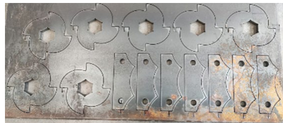
Figura 8 Corte por láser de material.
