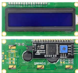
Figura 5 LCD I 2 C 16X2.
