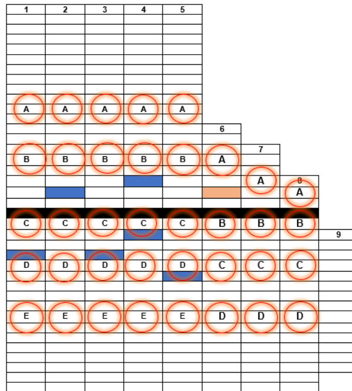
Figura 6 Plano del invernadero.
