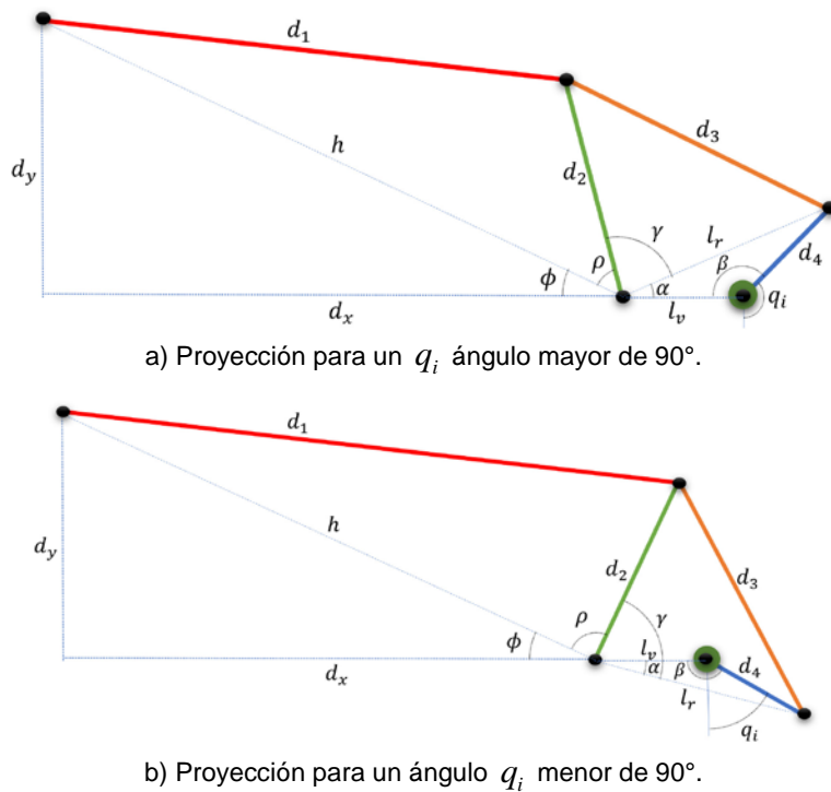
Figura 4 Proyección geométrica del mecanismo de 4 barras.
