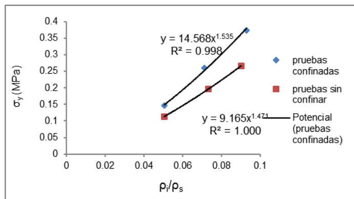
Fig. 9. Esfuerzo de fluencia como función de la densidad relativa.
