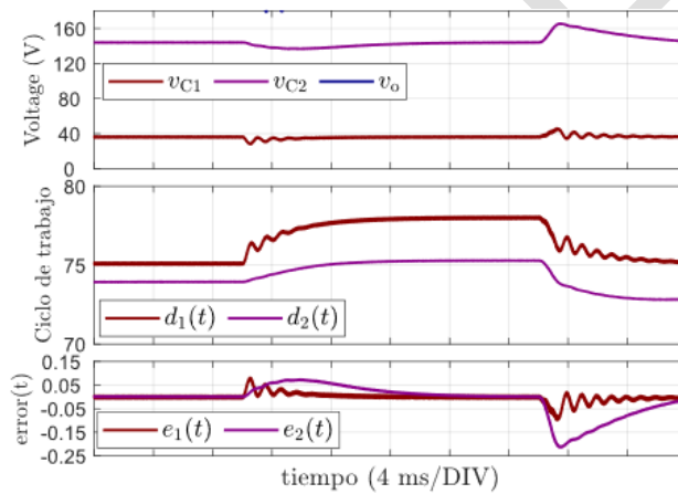
Figura 10 Comportamiento dinámico del controlador, bajo un cambio en la carga.
