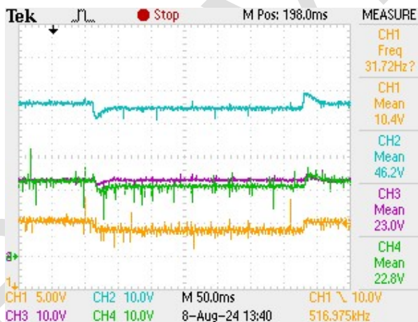
Figura 12 Respuesta de los controladores ante una disminución de voltaje de entrada.
