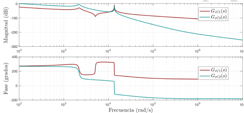
Figura 4 Diagramas de Bode de las funciones de G_{vC1}(s) y G_{vC2}(s) en lazo cerrado.
