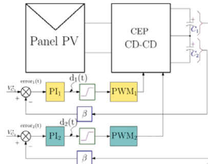
Figura 1 Diagrama de bloques de la estructura usada para la técnica propuesta.
