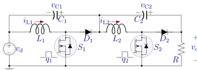
Figura 2 Topología del convertidor de potencia empleado para realizar el control híbrido.
