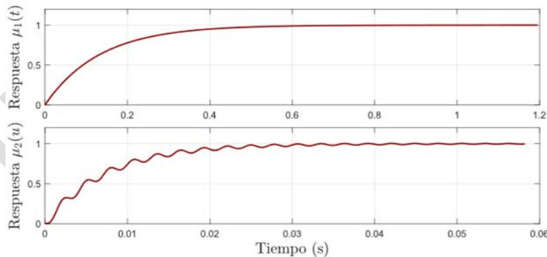
Figura 5 Respuesta ante una entrada escalón unitario.
