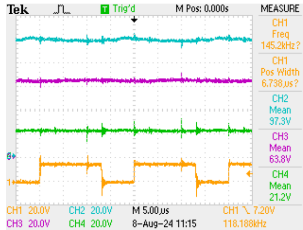
Figura 11 Formas de onda de la operación en estado estable del convertidor.
