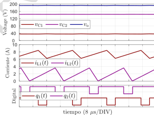
Figura 8 Formas de onda representativas del funcionamiento del CEP en estado estable.
