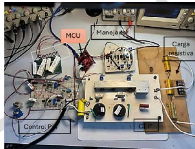
Figura 6 Prototipo de la topología del convertidor del tipo cuadrático.
