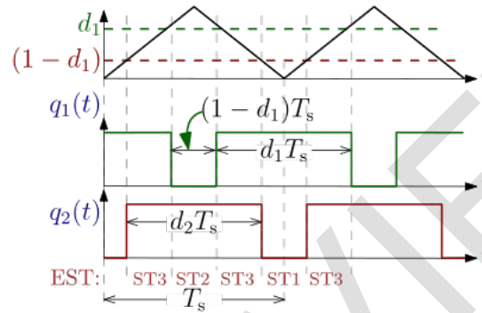
Figura 3 Estrategia de conmutación síncrona, en contrafase para cada transistor.
