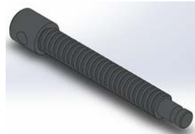
b) Tornillo de potencia AISI 4140 templado y revenido.
