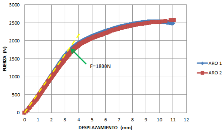
Fig. 8. Resultados experimentales (Fuerza vs desplazamiento), aro Ilizarov 180°-180 mm.
