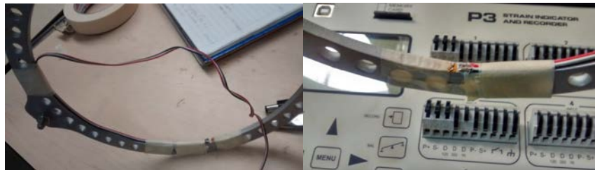
Fig. 19. Conexión e instrumentación.
