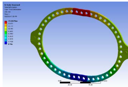
Fig. 12. Deformación total (mm).
