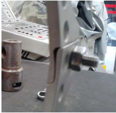
Fig. 9. Deformación de la unión atornillada del aro a carga máxima.
