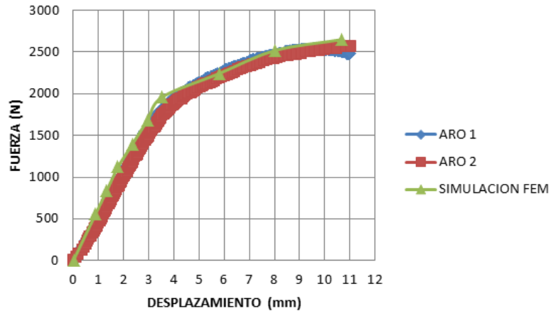
Fig. 16. Resultados experimentales (ARO 1 y ARO 2) versus simulación numérica.
