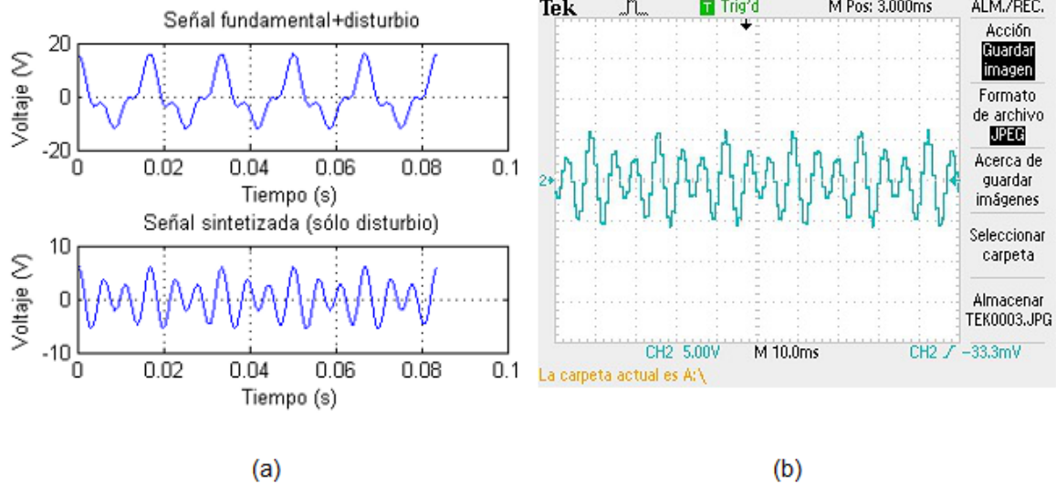
Fig. 11. Armónicos: (a) Simulación, (b) Señal física analógica.
